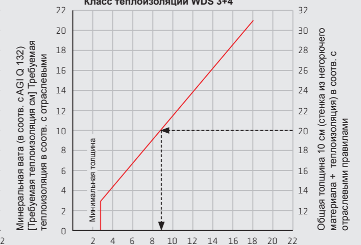
б) В качестве замены комбинированной теплоизоляционной стенки и теплоизоляции Класс теплоизоляции WDS 3+4
